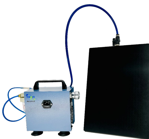
真空涂布台
